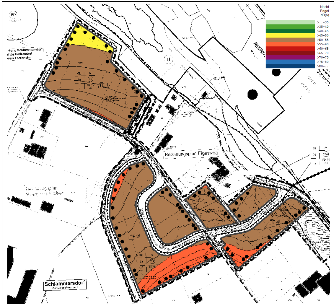
Abbildung 3: Beurteilungspegelkarte Anlagengeräusche, Beurteilungszeitraum nachts, Aufpunkthöhe h = 12\text{ m} ü. Gel.
